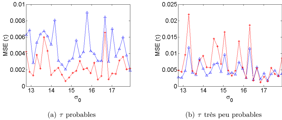
FIG. 2.5 – Comparaison des MSEs en fonction de \sigma_0 : *— MCMC et —△— MLE
