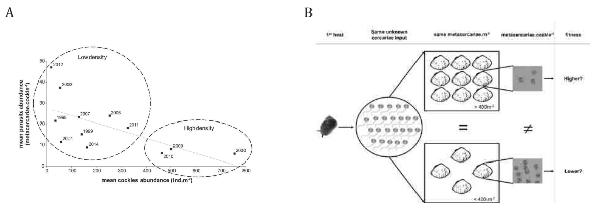
Figure 5 A. Nombre moyen de parasites par coque en fonction de la densité moyenne annuelle des coques (adultes). B. Schéma conceptuel illustrant l'hypothèse selon laquelle, à quantité de parasites constant, la densité des coques influe sur l'infestation individuelle. Magalhães et al. 2016.
