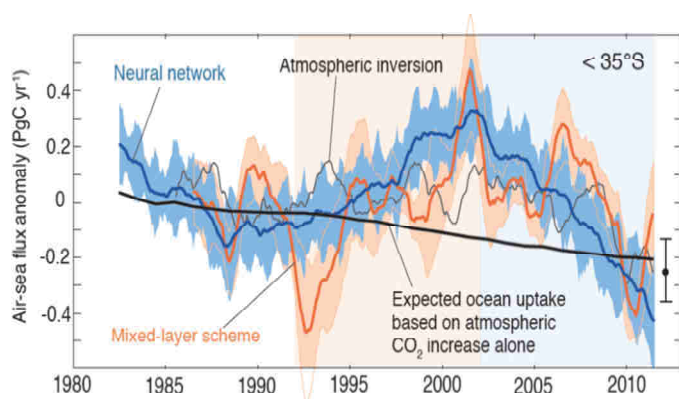
Figure 9 : Variabilité des Flux de CO 2 air-mer dans l'océan Austral, sur la période 1982-2011 évaluée par une Inversion Atmosphérique (grisé) et 2 méthodes (bleu et orange) basées sur la base SOCAT (Landschützer et al., 2015). La tendance liée uniquement à l'augmentation de CO 2 atmosphérique, sans prendre en compte la variabilité climatique, est également indiquée en noir
