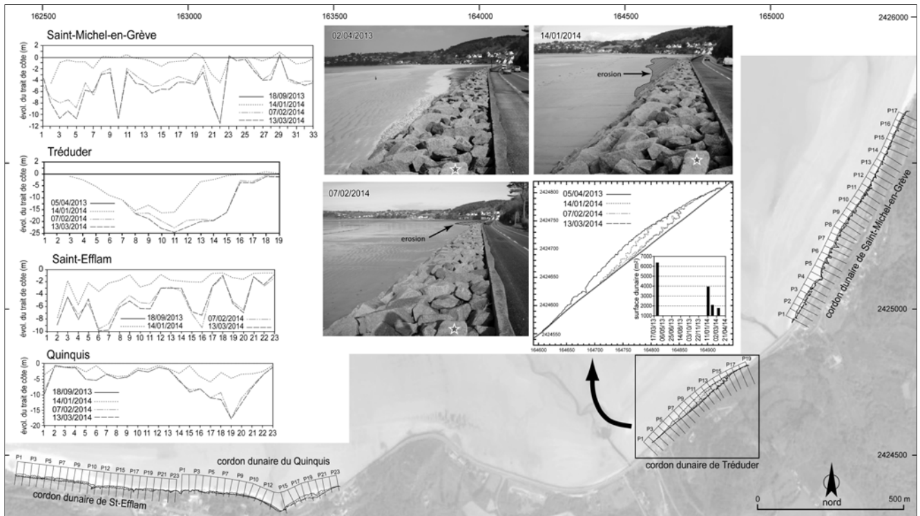
Fig. 8 – Illustration des trois phases de recul du trait de côte de la baie de Saint-Michel-en-Grève (Côtes d'Armor).
