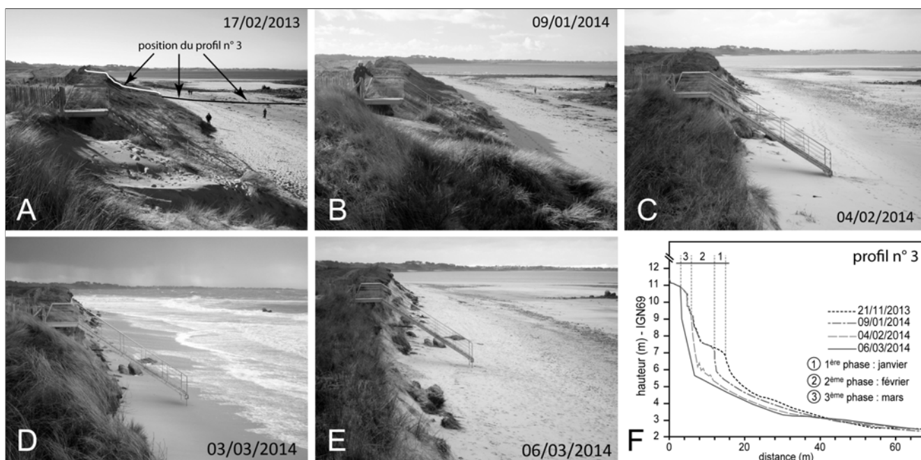
Fig. 7 – Illustration des trois phases de recul du trait de côte pour le cordon littoral sableux de la plage du Vougot (Guissény – nord Finistère).
