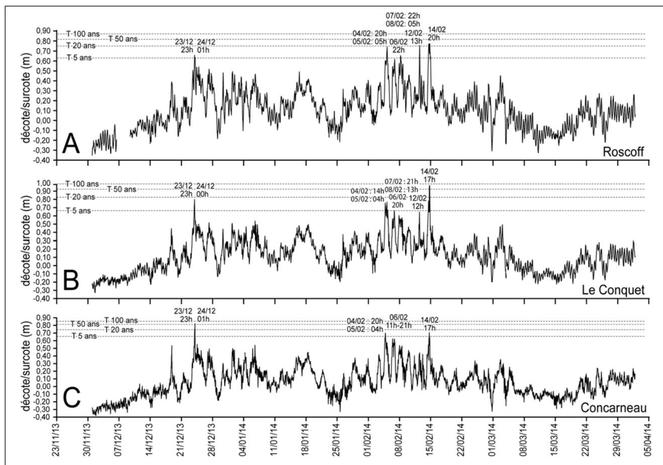
Fig. 4 – Analyse des surcotes enregistrées par les marégraphes de Roscoff pour la côte nord de la Bretagne (A), du Conquet pour la pointe occidentale (B), et de Concarneau pour la côte méridionale (C), comparées aux niveaux de surcote maximum pour des périodes de retour de 5, 20, 50 et 100 ans.
