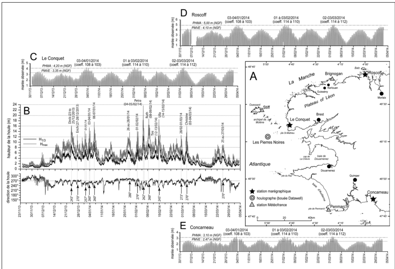
Fig. 3 – Caractéristiques de la houle basée sur les enregistrements réalisés au large du Finistère par la bouée Datawell des Pierres Noires, et marées observées pour la côte nord, ouest et sud de la Bretagne, entre les mois de décembre 2013 et mars 2014. A : localisation de la bouée Datawell des Pierres Noires et des marégraphes de Roscoff, du Conquet et de Concarneau ; B : hauteurs et directions de la houle. Marée observée au Conquet (C), à Roscoff (D), à Concarneau (E), comparée au niveau des pleines mers de vive-eau et au niveau des plus hautes mers astronomiques.
