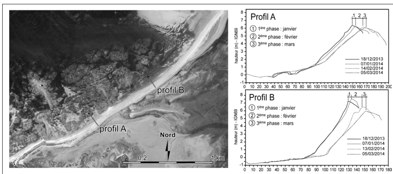
Fig. 10 – Illustration des trois phases de recul du trait de côte par rollover de la flèche de galets du Sillon de Talbert (Côtes d'Armor).
