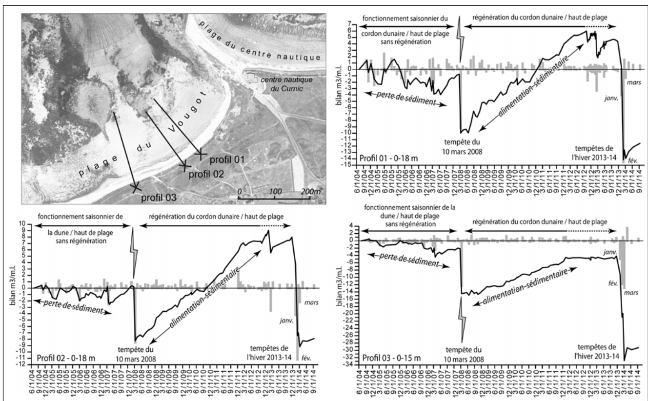
Fig. 14 – Evolution du bilan sédimentaire du cordon dunaire de la plage du Vougot (Guissény) dans sa partie orientale entre les mois de juin 2004 et septembre 2014.
