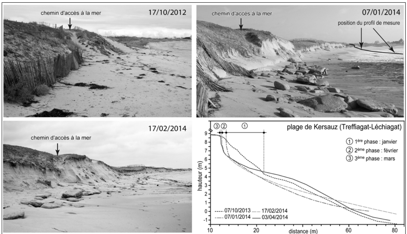
Fig. 9 – Illustration des trois phases de recul du trait de côte pour le cordon littoral sableux Treffiat-Léchiagat (sud Finistère).
