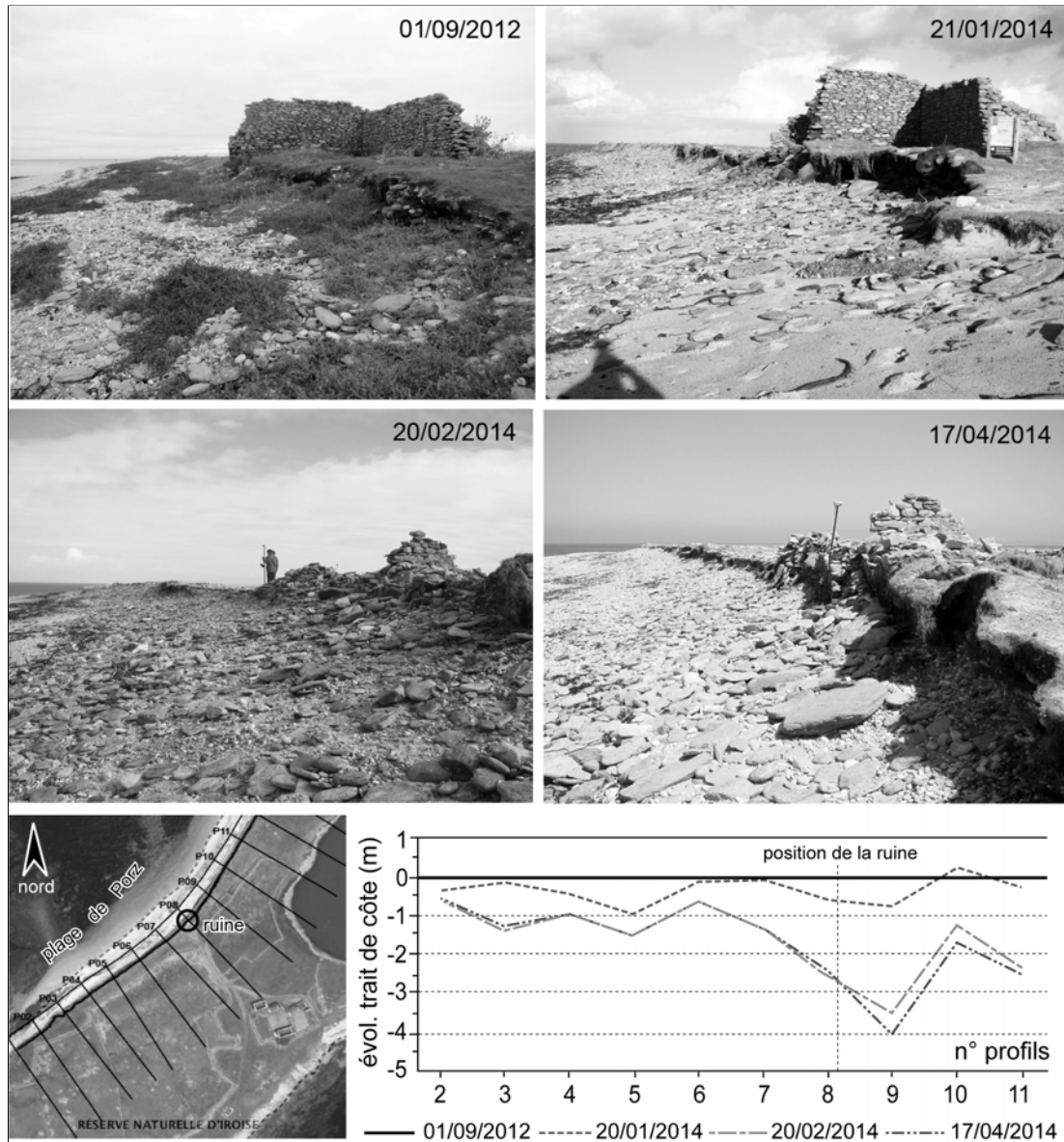
Fig. 11 – Illustration des trois phases de recul du trait de côte du cordon de galets de la plage de Porz sur l'île de Triélen – archipel de Molène (ouest Finistère).
