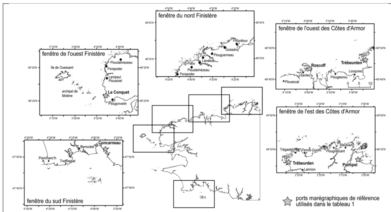
Fig. 1 – Localisation des fenêtres de calcul des paramètres statistiques de houle issues du modèle PREVIMER (source : http://www.previmer.org )
