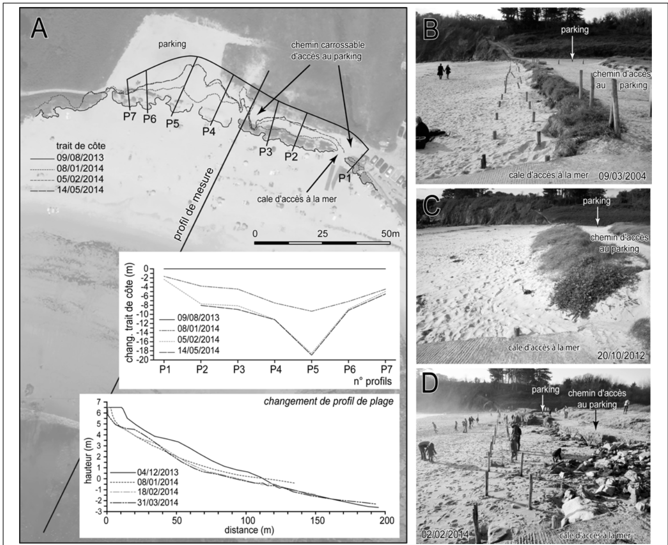
Fig. 13 – Erosion du trait de côte et destruction des aménagements littoraux de la plage de Porsmilin – ouest Finistère. A : Variation du trait de côte et changement de profils de plage ; B : situation avant les tempêtes le 09/03/2004 ; C : le 29/10/2012 ; D : situation après tempête le 02/02/2014.
