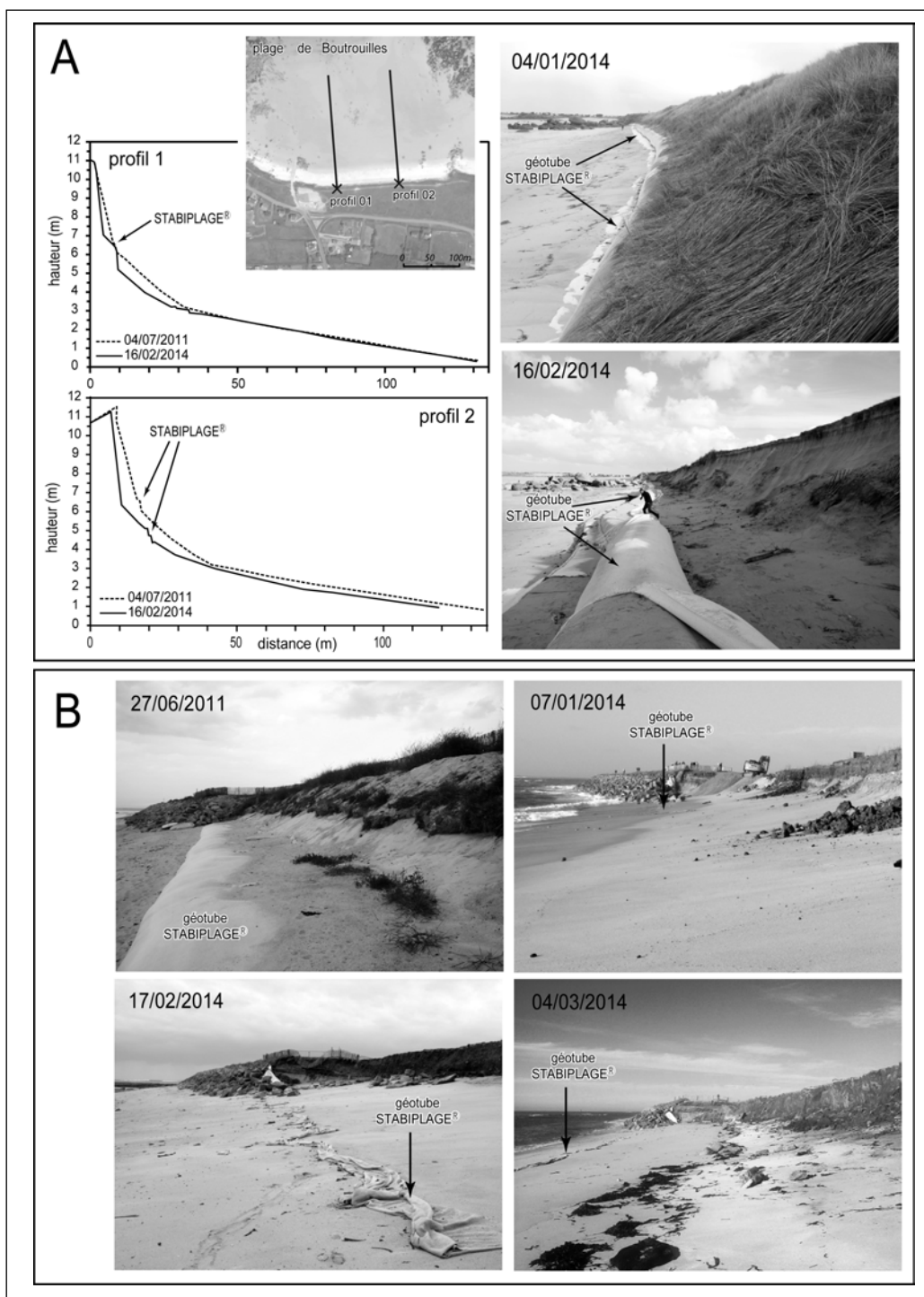
Fig. 12 – Erosion du trait de côte et destruction des ouvrages de défense du littoral de la plage Boutrouilles à Kerlouan – nord Finistère (A), et de la plage de Léhan à Treffiagat-Léchiagat – sud Finistère (B).
