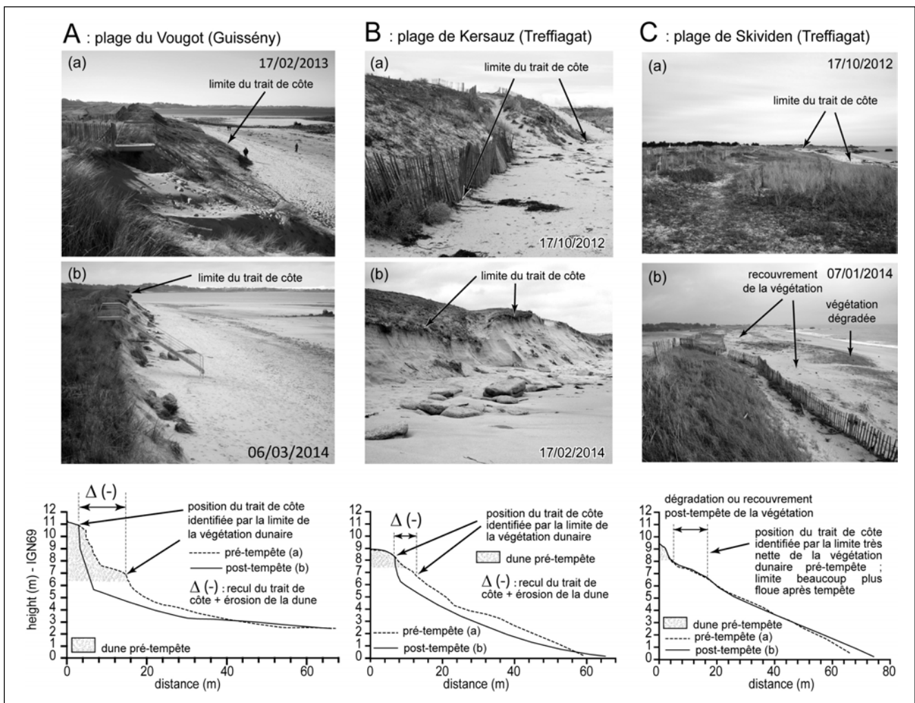
Fig. 5 – Approche méthodologique suivie pour la définition d'une limite bio-morphologique du trait de côte. A : exemple d'un cordon dunaire dont tout le versant externe a reculé ; B : exemple d'un cordon dunaire dont seule une partie du versant externe a reculé ; C : exemple d'un cordon dunaire partiellement submergé sans qu'il n'y ait de recul de l'édifice.
