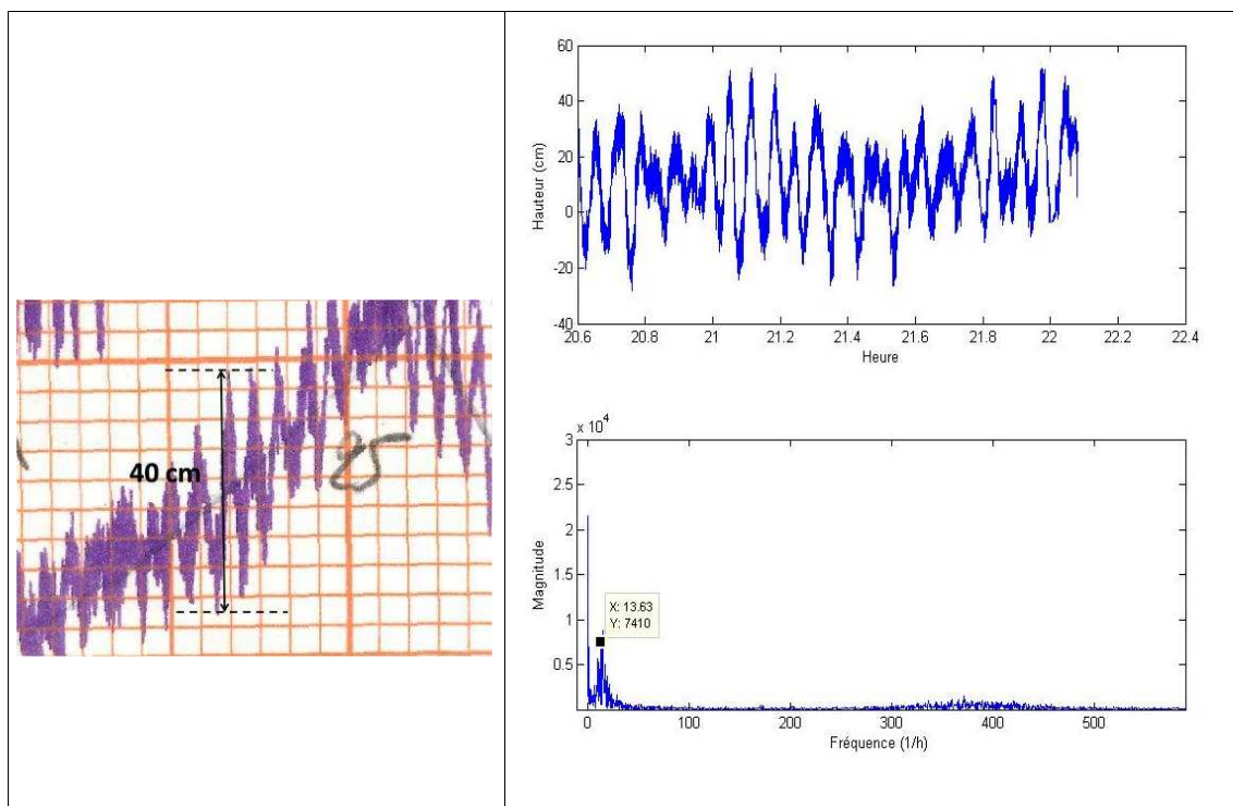
Figure 1. A gauche: illustration de l'estimation de la hauteur de seiche à Port-Tudy (cas du 25 février 2007). A droite: Signal (en haut) et spectre (en bas) de seiche (Port-Tudy, 16 janvier 2008).
