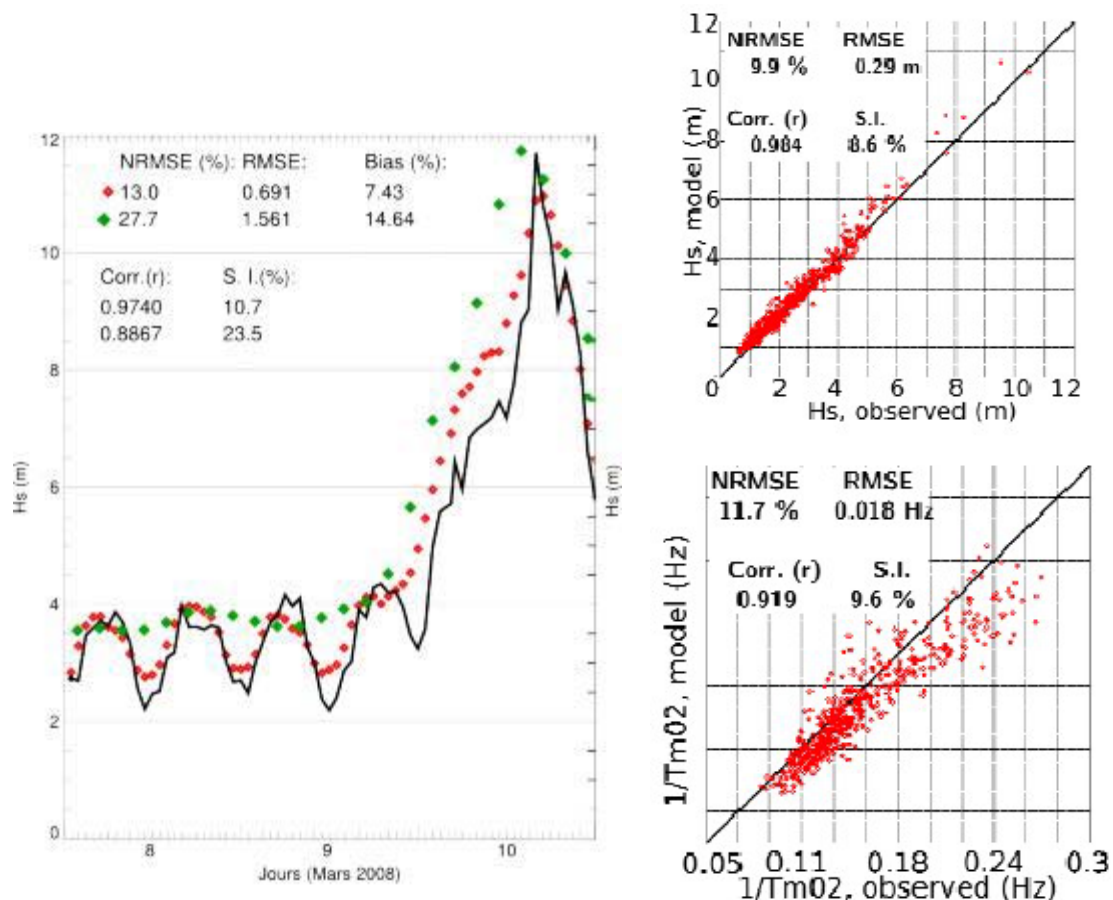
Figure 3. A gauche: comparaison entre H_s mesuré par la bouée des Pierres noires (courbe noire) et les modélisations avec (petits symboles rouges) et sans (gros symboles verts) prise en compte des courants. A droite: comparaison modèle-mesure avec des mesures moyennées sur 3 h, pour la hauteur des vagues (en haut) et la fréquence moyenne (en bas), de janvier à mars 2008.
